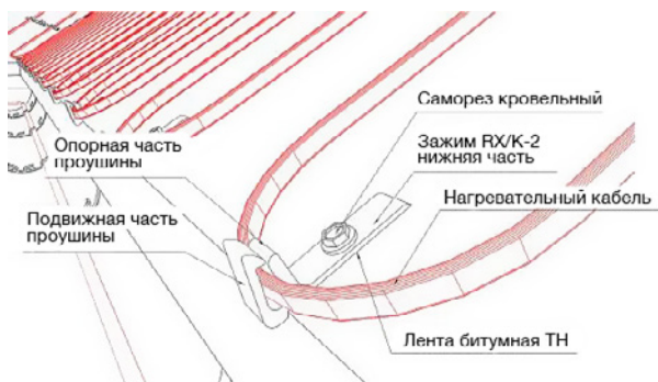
Рис. 4 (Зажим РХ/К-2)
